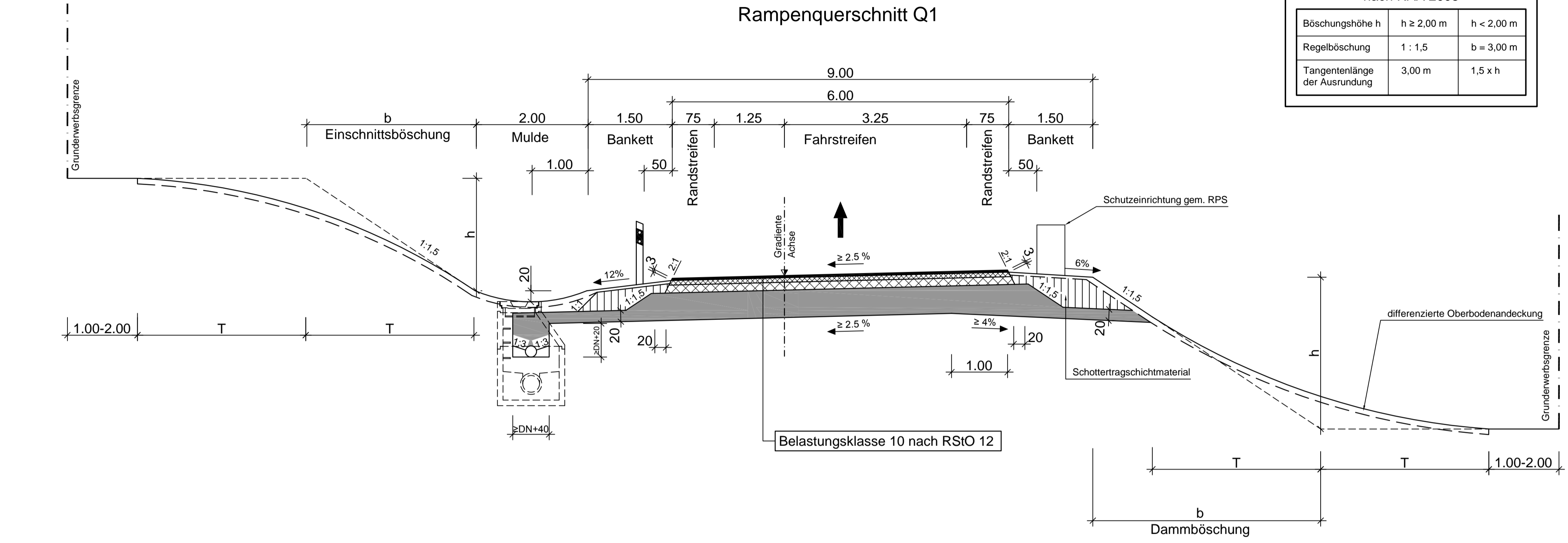
Rampenquerschnitt Q4
